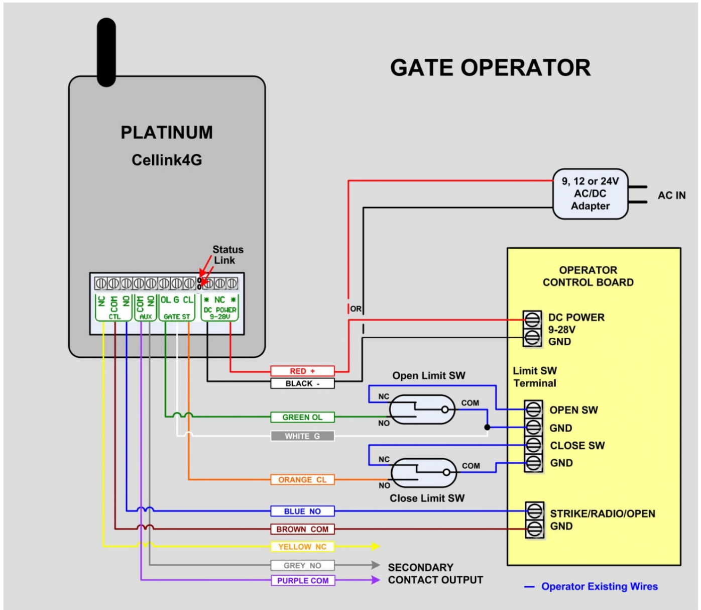
Fig. 4 Wiring Diagram
